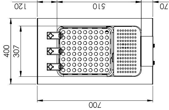
Draufsicht / Top view
