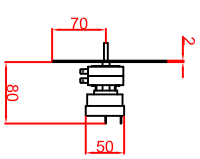
Einbauleite Thermostat 85mm
