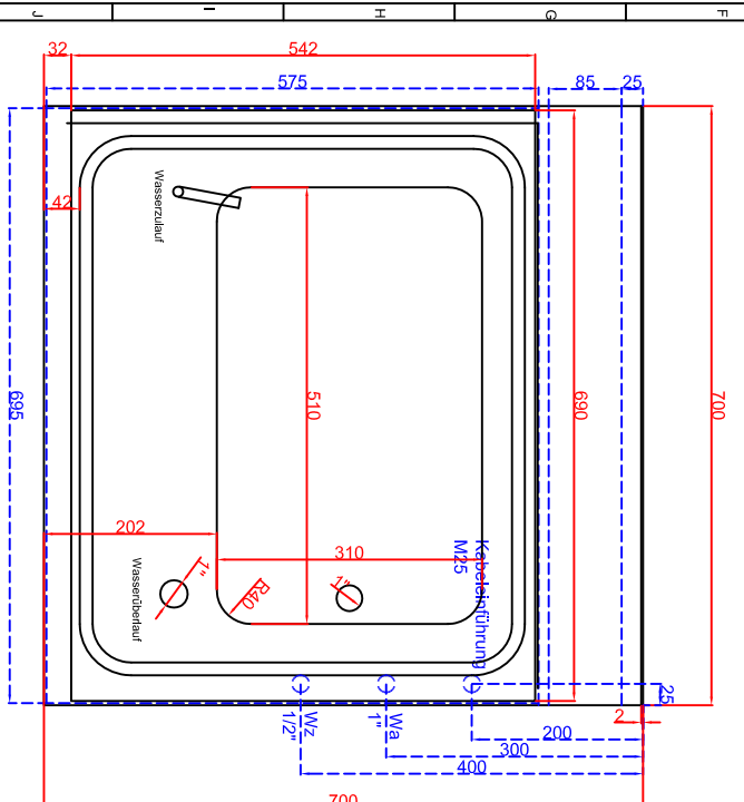
Draufsicht
