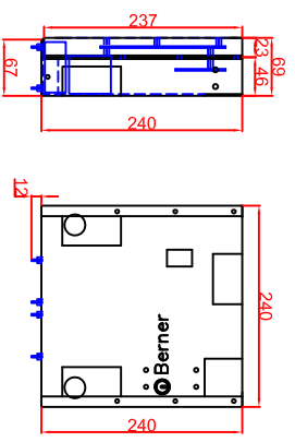
Generatoransichten Version Generator-Spule getrennt Seitenansicht Frontansicht
