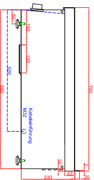
Seitenansicht
