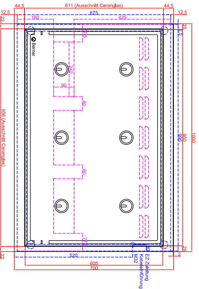
Draufsicht
