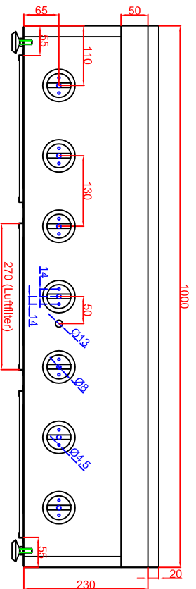
Frontansicht
