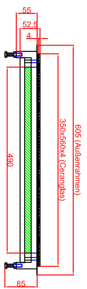
Ausschnitt in Abdeckung flächenbündiger Einbau 356mm x 566mm
