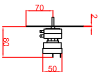
Einbauliste Thermostat 85mm
