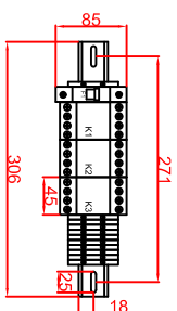
Platz für Schaltung in Unterbau vorsehen
