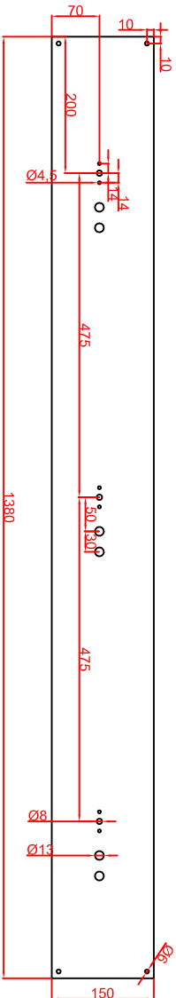
Schalterblende (optional lieferbar)
