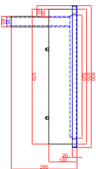
Seitenansicht
