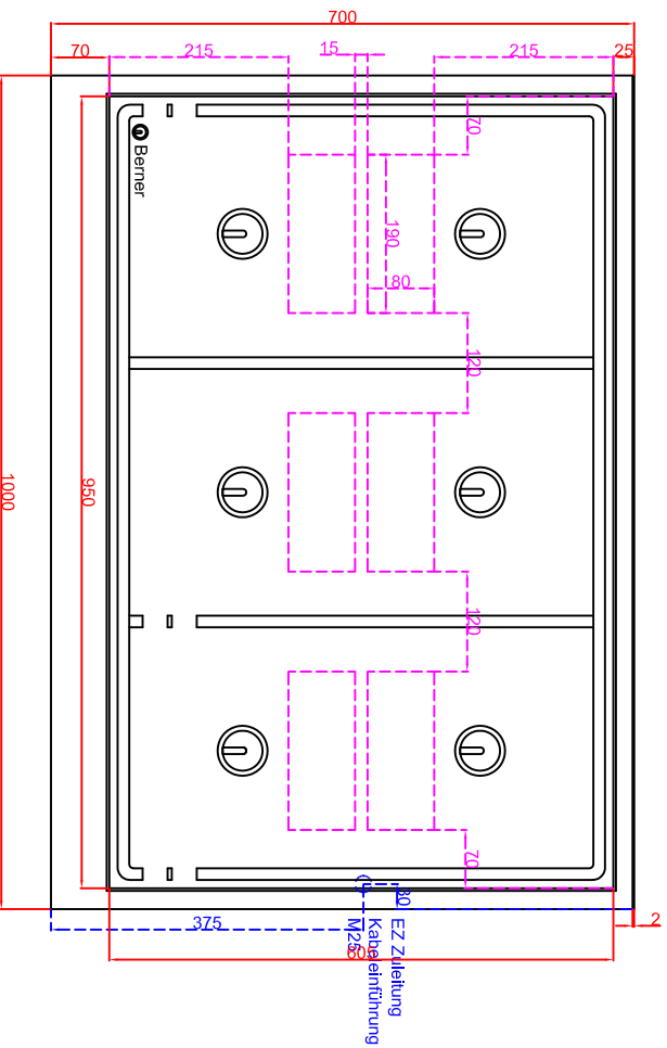
Draufsicht
