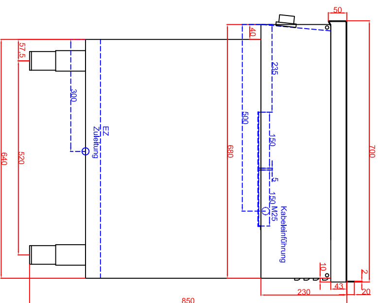
Seitenansicht
